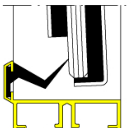
Höhenschnitt M=1:1
