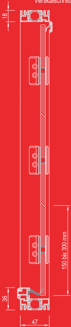
Vertikalschnitt
