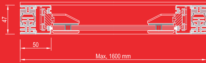
Vertikalschnitt
